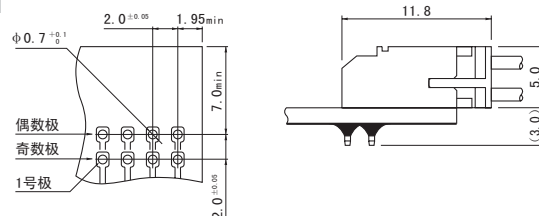
侧装型
