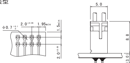
顶装型
